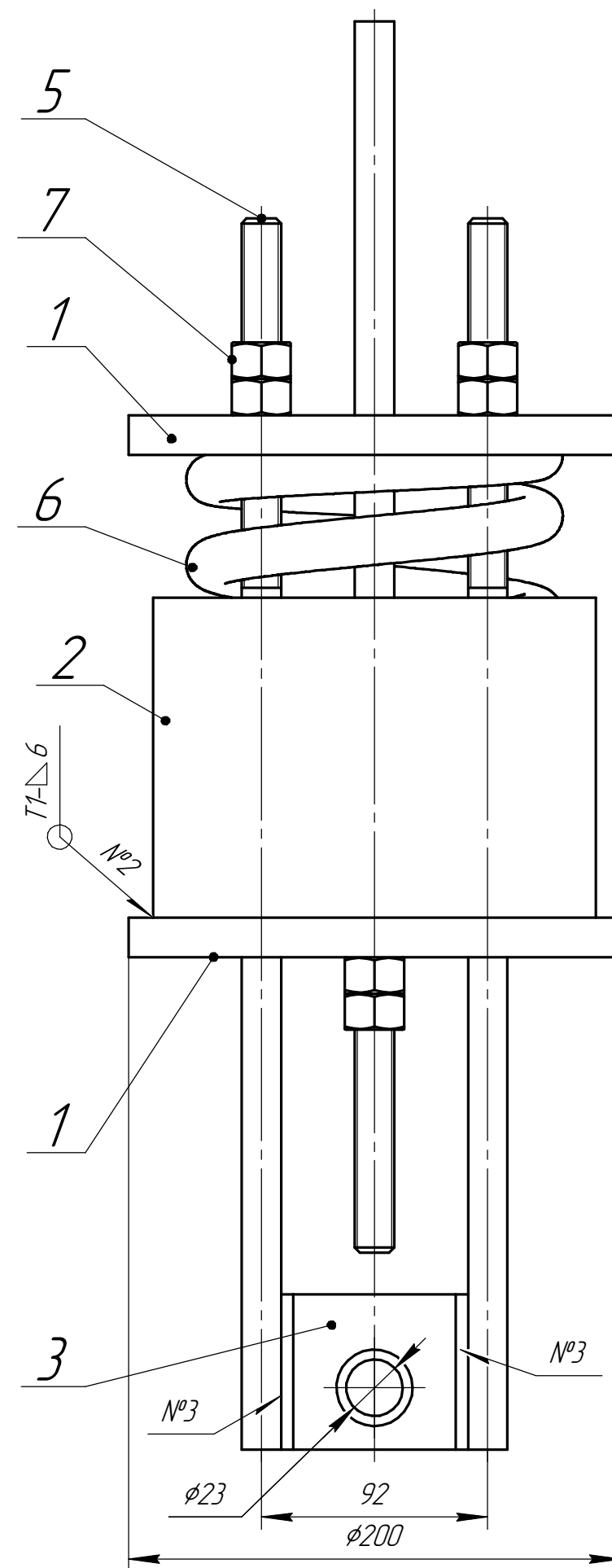
A-A(1:1)
