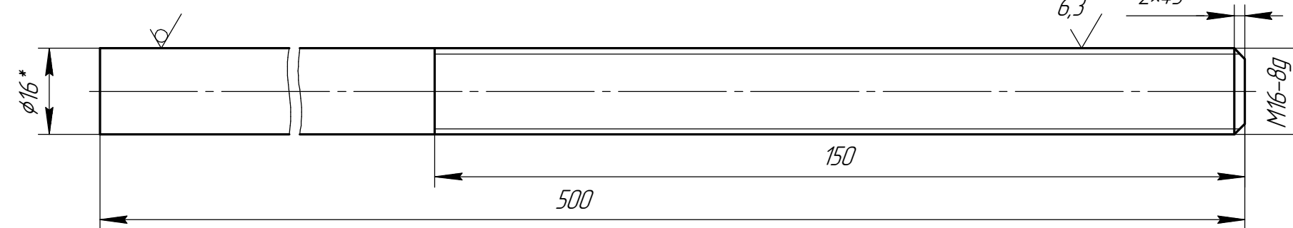
Дет. поз. 5 (1:1)
