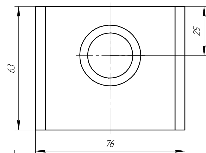
Дет. поз. 3 (1:1)
