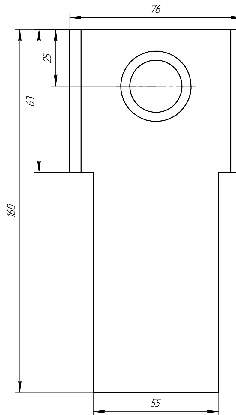
Дет. поз. 4 (1:1)
