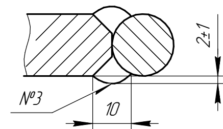
A-A(1:1)
